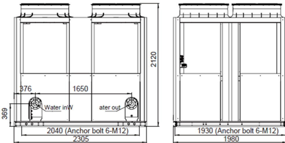
LSQWRF130VM/NhA-M (Unit:mm)
